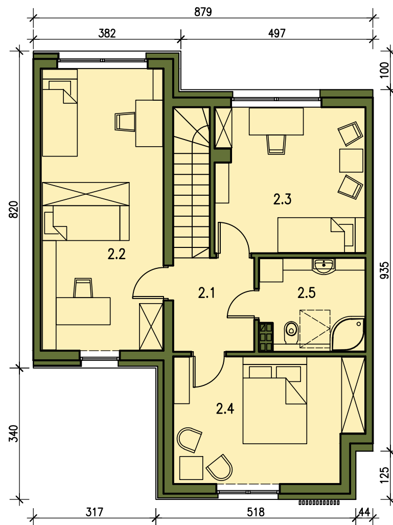
RZUT PIĘTRA
