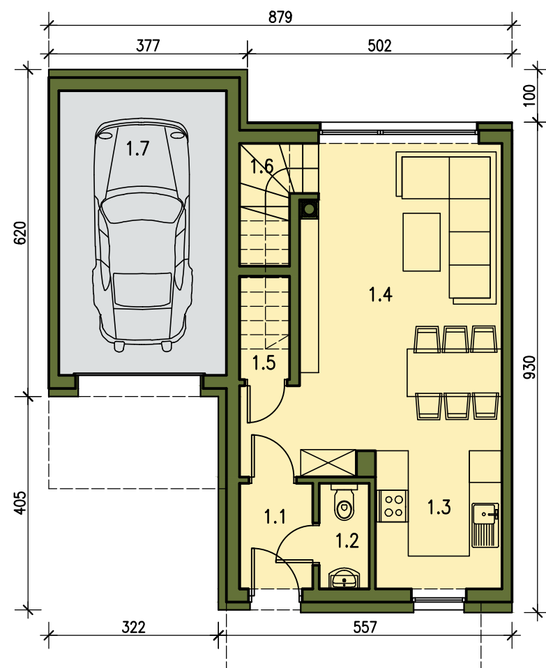
RZUT PARTERU
