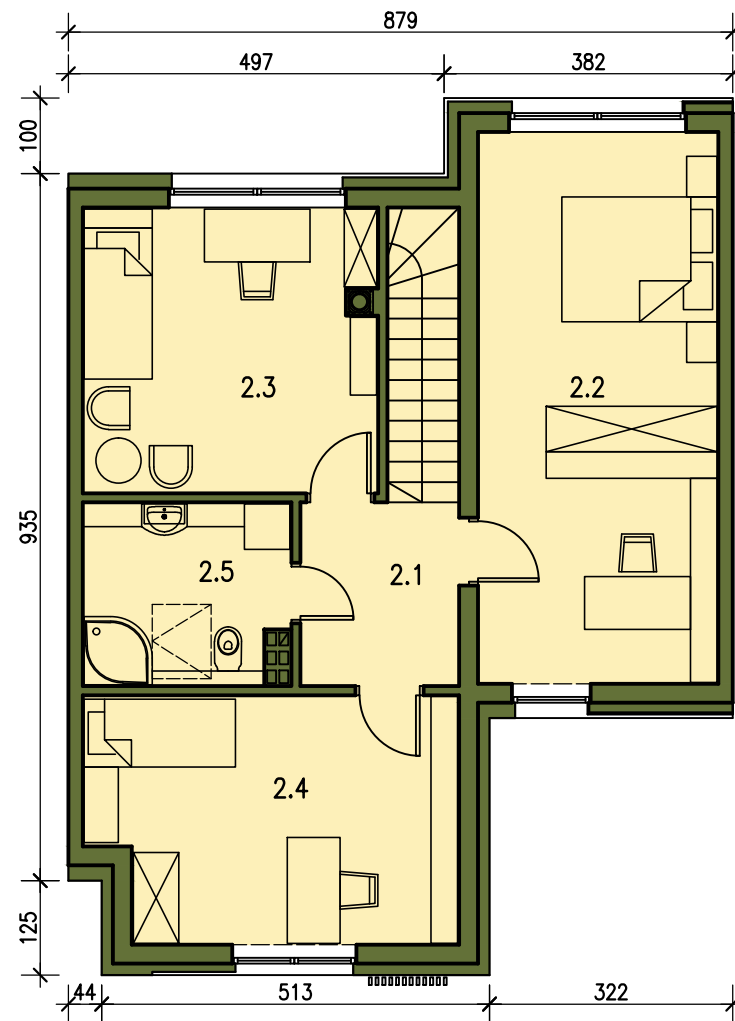
RZUT PIĘTRA
