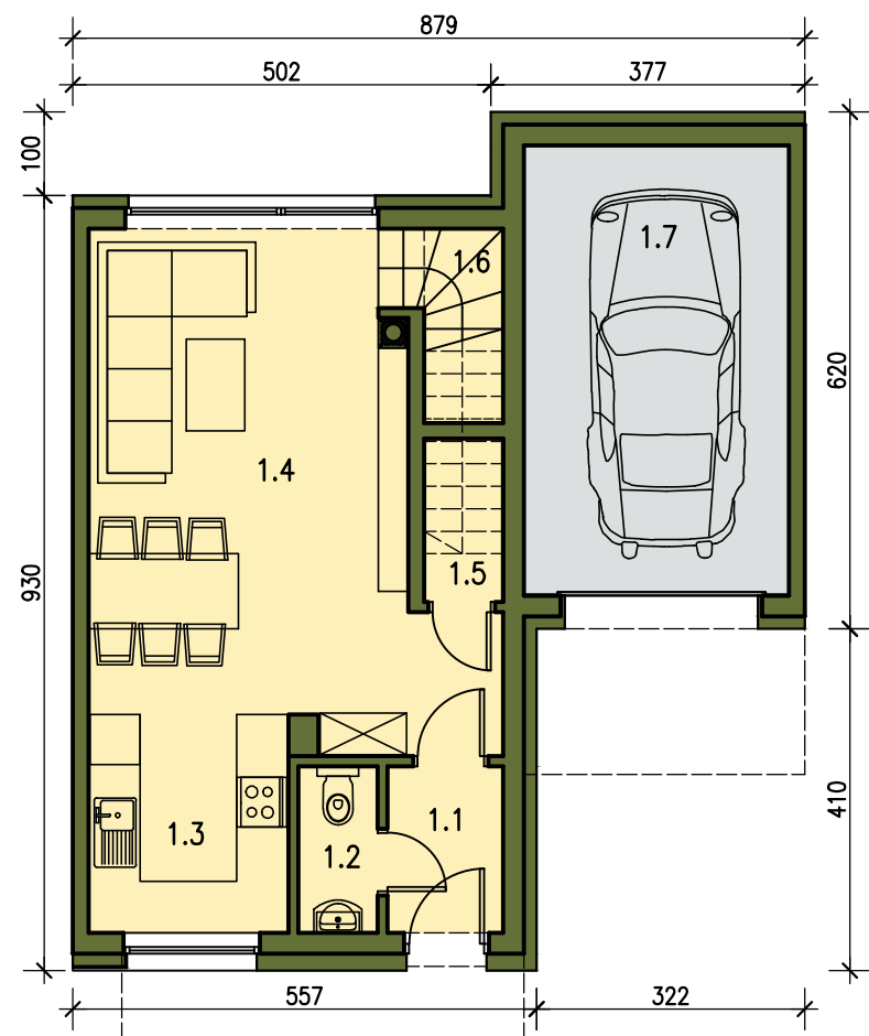
RZUT PARTERU
